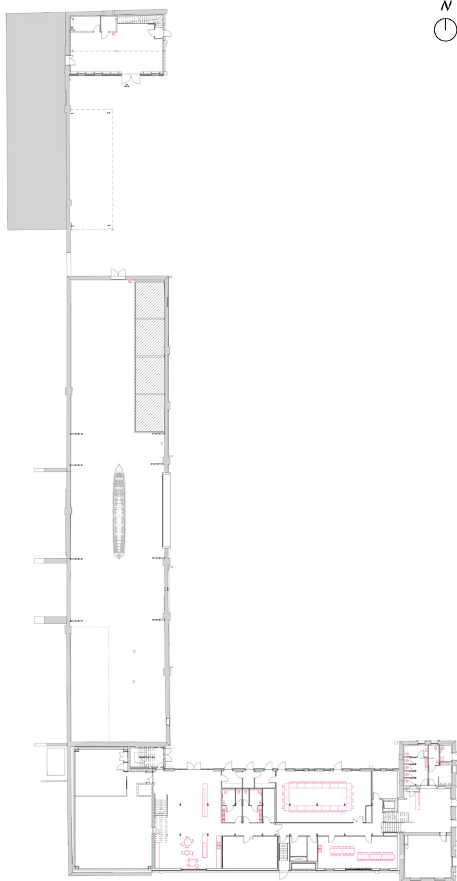
18 - Plan rdc
